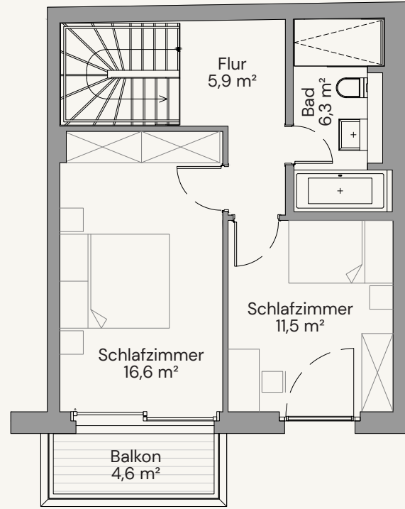
1. Obergeschoss | 1 st floor
