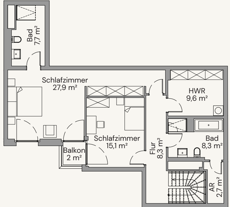
1. Obergeschoss | 1 st floor
