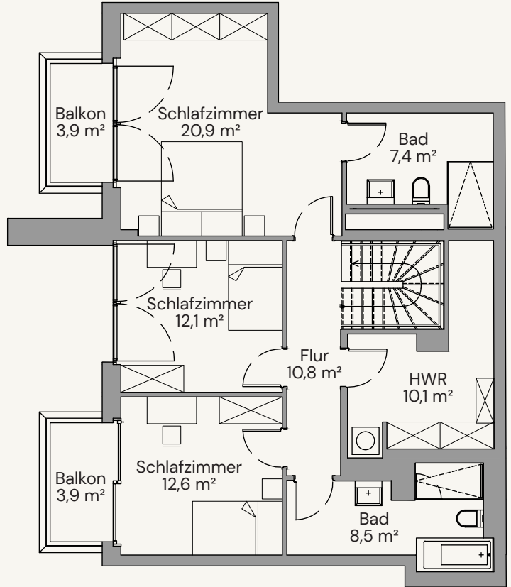
1. Obergeschoss | 1 st floor
